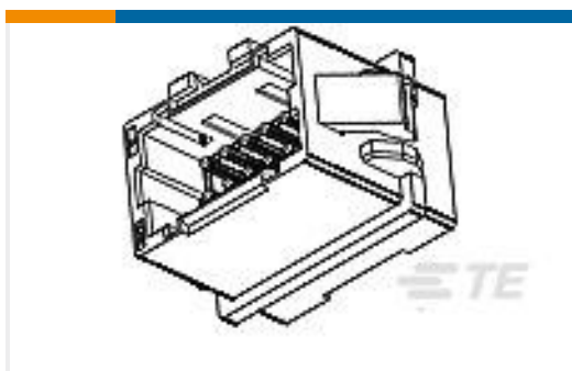
TE Part #2-292216-6 MINI CT D/R RELAY 26P V NAT
