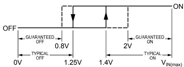
Enable Hysteresis
