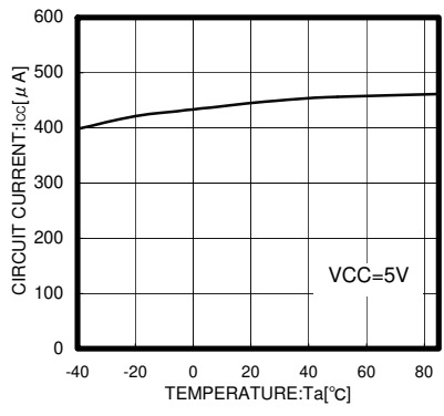
Fig.13 Ta - Icc
