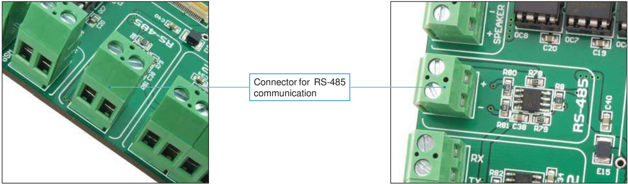
Figure 7-1: RS-485 module
