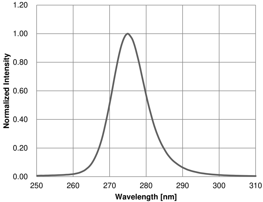
Fig 1. Spectrum, T_a=25^\circ\text{C} , I_F=150\text{mA}
