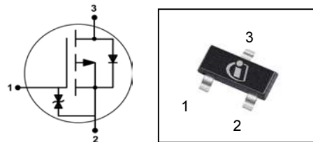
PG-SOT-23
