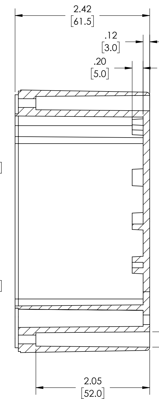
SECTION A-A
