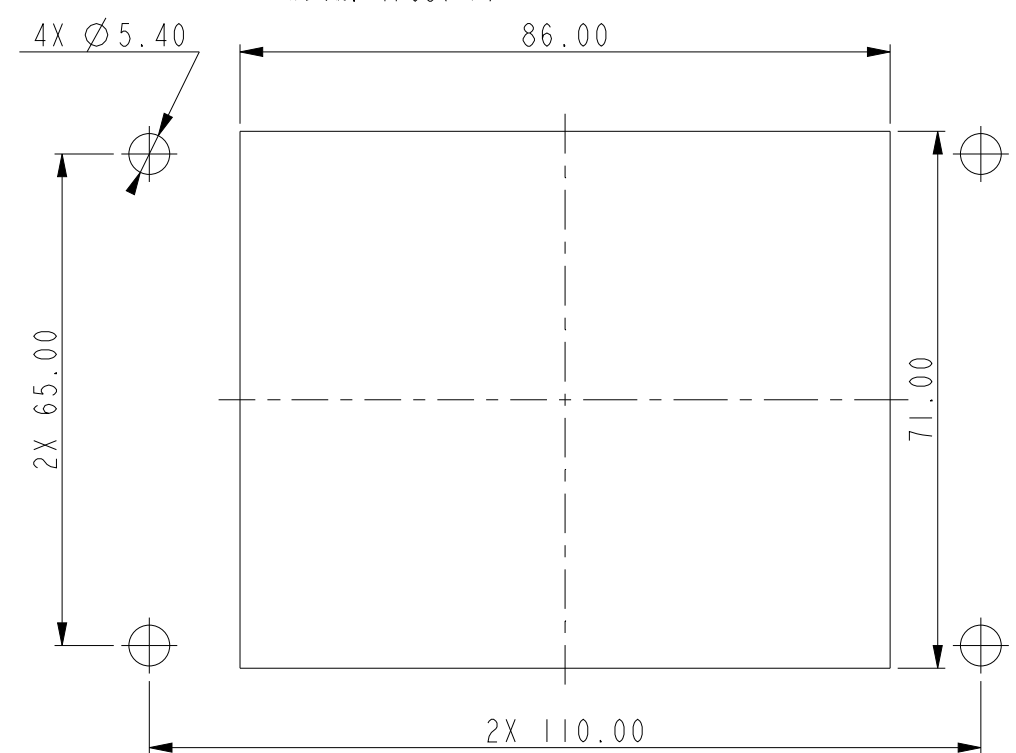
开孔安装示意图 PANNEL CUT OUT
