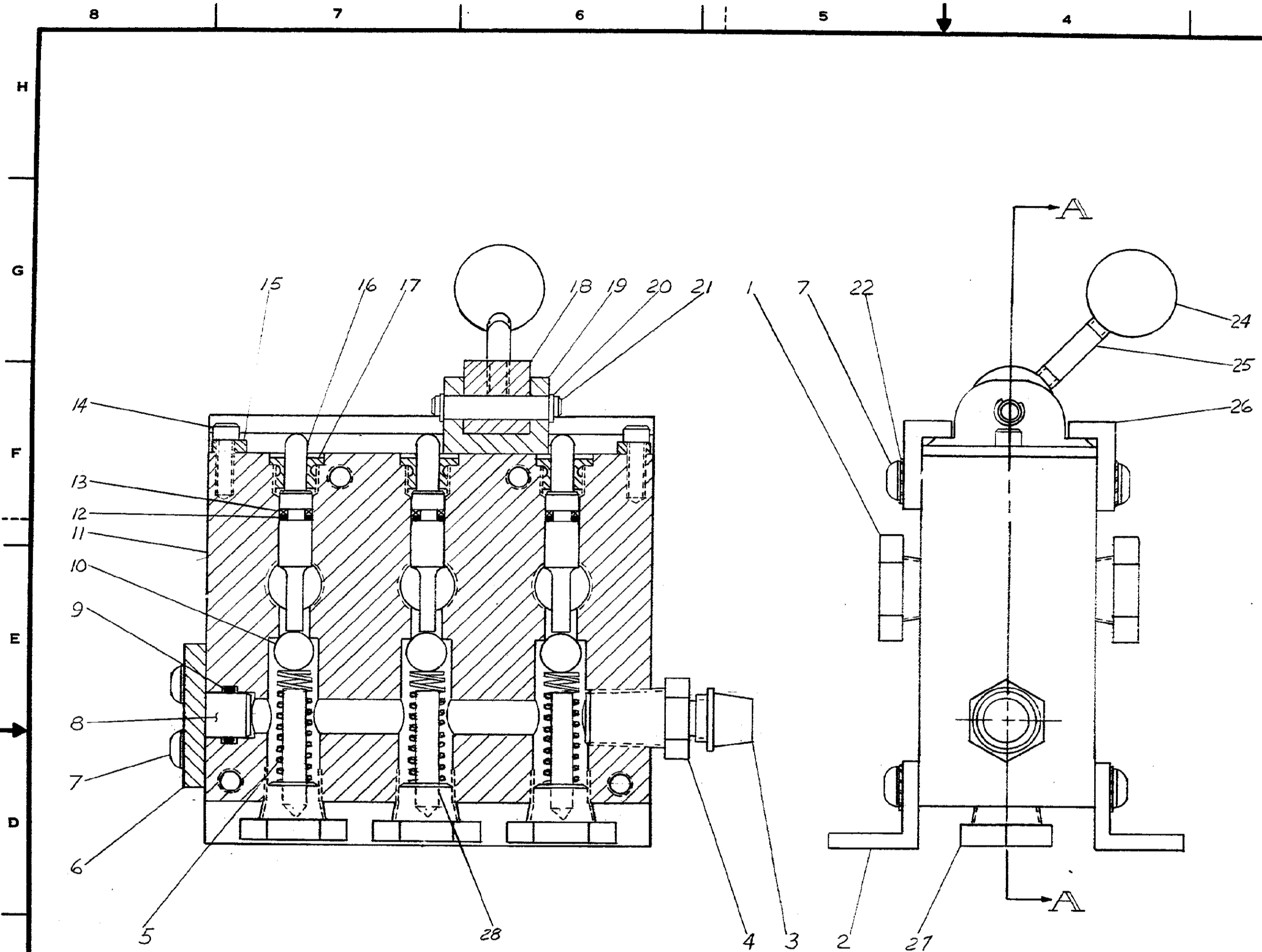
SECTION A-A
