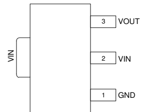
SOT89
