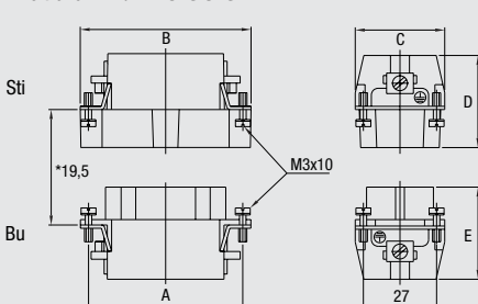
Maßbild mm/Dimensions mm
