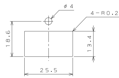
PANEL CUT OUT DIMENSION (REF.) パネル開口寸法 (参考)
