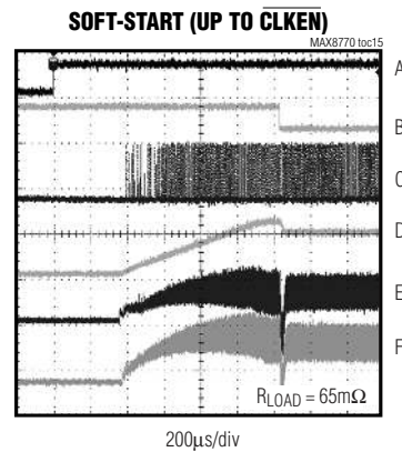
A. \overline{SHDN} , 5V/div B. \overline{CLKEN} , 10V/div C. I_{LX1} , 10V/div D. V_{OUT} , 1V/div E. I_{LX1} , 10A/div F. I_{LX2} , 10V/div
