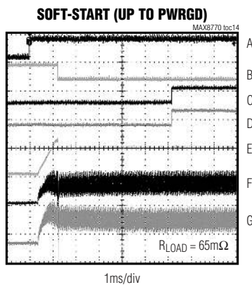
A. \overline{SHDN} , 5V/div B. \overline{CLKEN} , 10V/div C. \overline{PWRGD} , 10V/div D. \overline{PHASEGD} , 10V/div E. V_{OUT} , 1V/div F. I_{LX1} , 10A/div G. I_{LX2} , 10V/div
