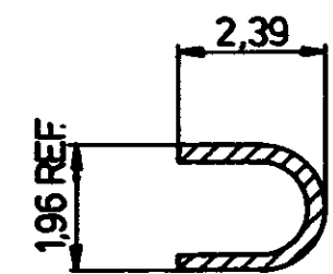
SCHNITT C-D
