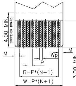
Section A-A Scale 2:1
