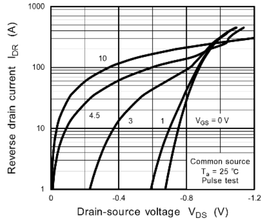
Fig. 8.6 I_{DR} - V_{DS}
