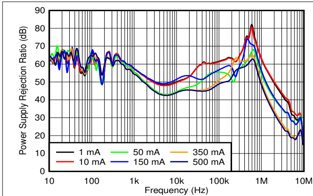
Figure 8-9. PSRR
