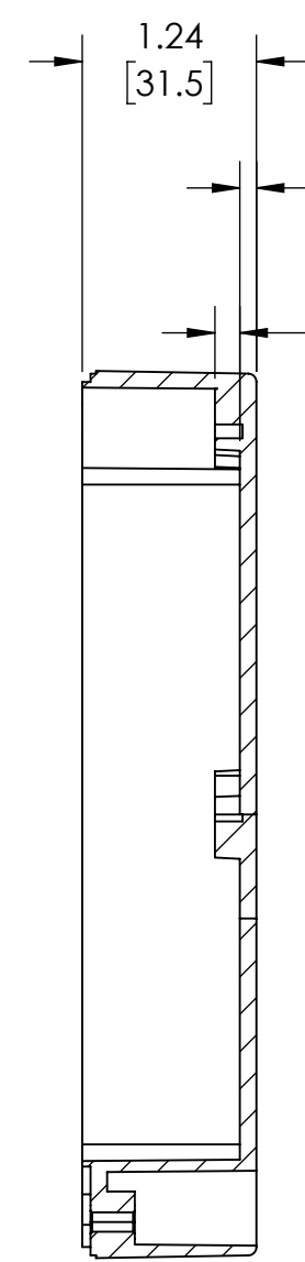
SECTION A-A SCALE 1 : 1.5
