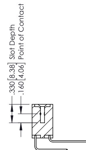
SECTION A-A
