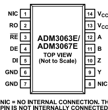
Figure 13. ADM3063E/ADM3067E 14-Lead SOIC_N Pin Configuration
