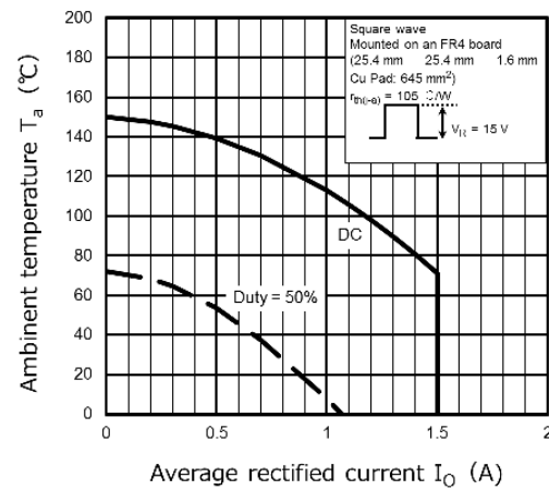
Fig. 8.6 T_a - I_O
