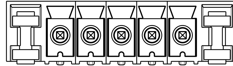
5 POLES: 2213933-5
