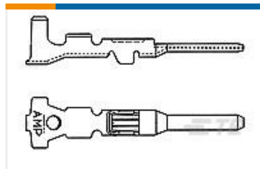
TE Part #282465-1 MINI MIC TAB CONTACT >1,5-
