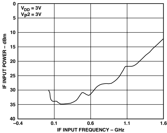
TPC 20. IF Input Sensitivity
