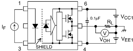
Fig. 13.1.3 V_{OH} Test Circuit
