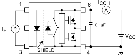
Fig. 13.1.5 I_{CCH} Test Circuit
