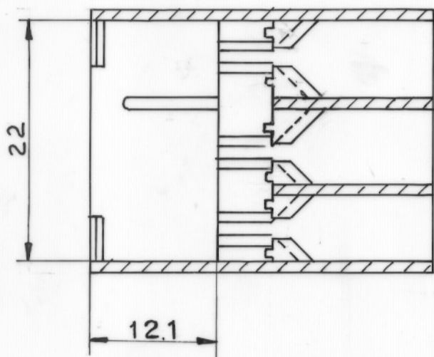
Sez. B-B
