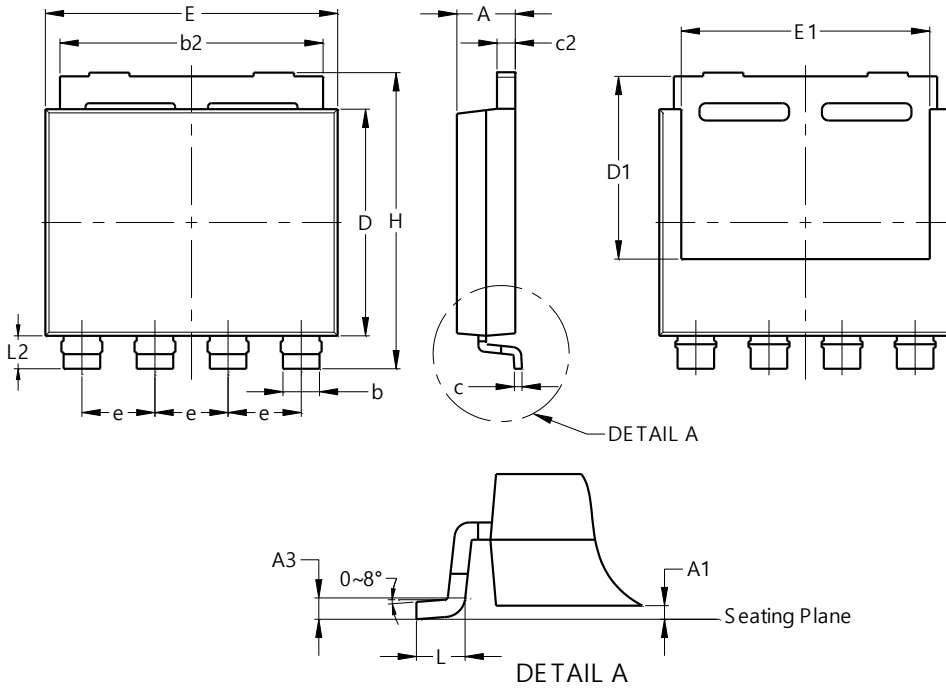
PowerDI8080-5
