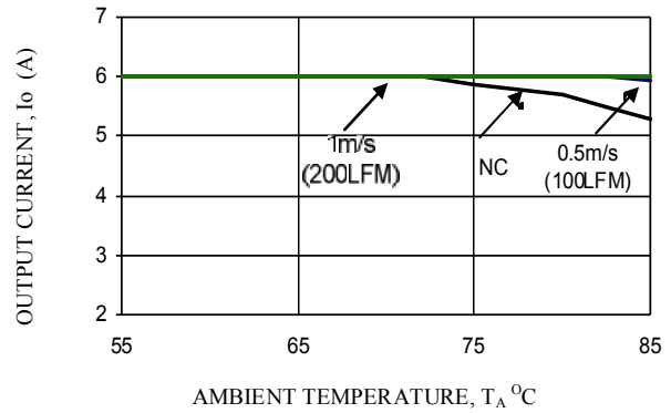
V_o=2.5V
