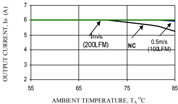
V_o=3.3V
