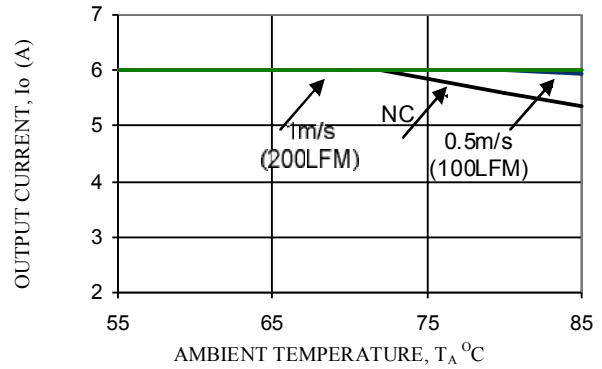
V_o=1.2V
