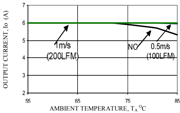
V_o=1.8V
