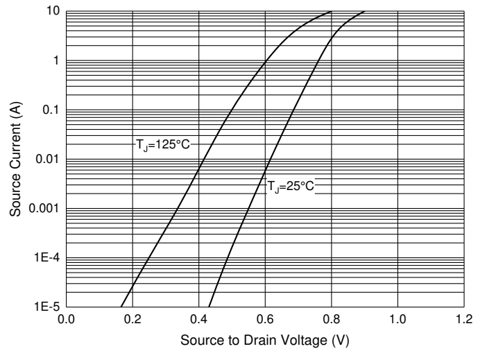
Fig. 4 - I_S - V_{SD}
