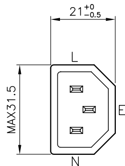
PLUG: COX-04
