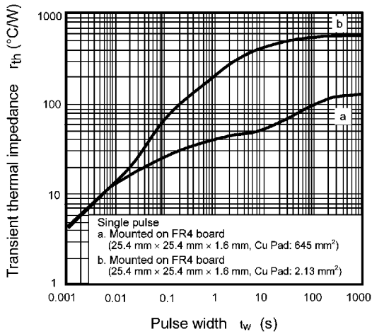
Fig. 7.13 r_{th} - t_w
