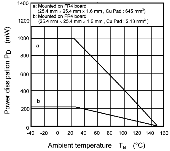
Fig. 7.14 P_D - T_a
