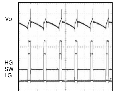
Fig.9 SLLM™ : I_o=1A
