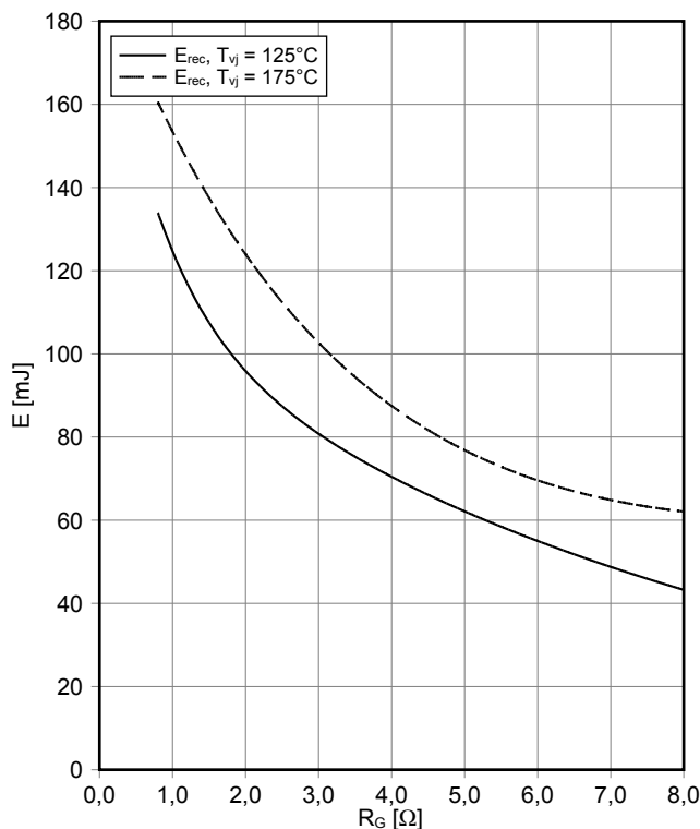
Schaltverluste Diode, Wechselrichter (typisch) switching losses Diode, Inverter (typical) E_{rec} = f(R_G) I_F = 1500 A, V_{CE} = 600 V
