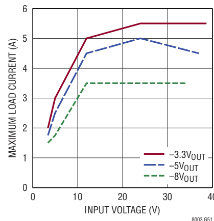
Maximum Load Current vs VIN \text{BIAS} Open
