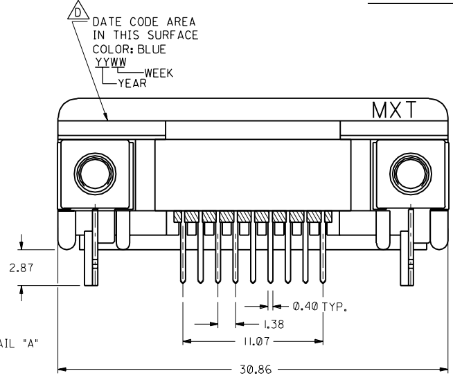
SCALE : 2 : 1
