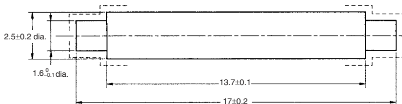
Actuator Dimensions
