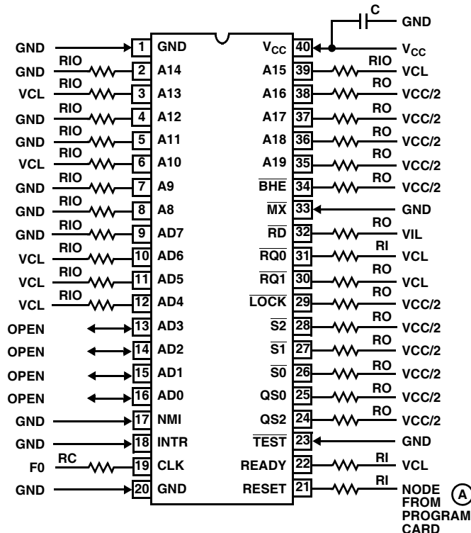
MD80C88 (CERDIP)
