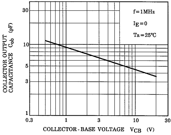
C_{ob} - V_{CB}
