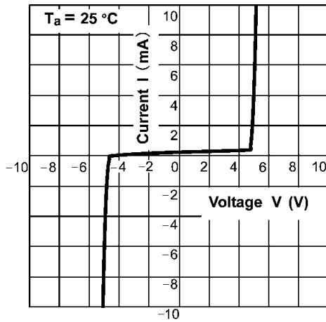
Fig. 7.1 I - V
