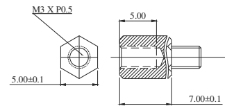
Hex Standoffs SCALE:3/1
