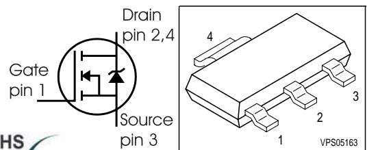
PG-SOT223
