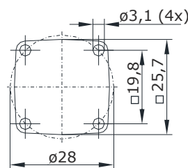
Hauptabmessungen Flansch
