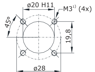
Montagefenster
