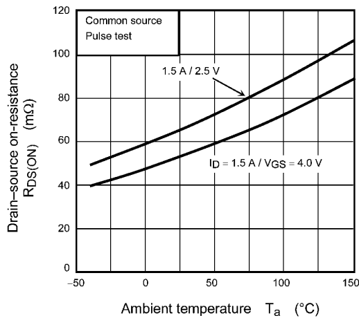
Fig. 7.1.5 R_{DS(ON)} - T_a
