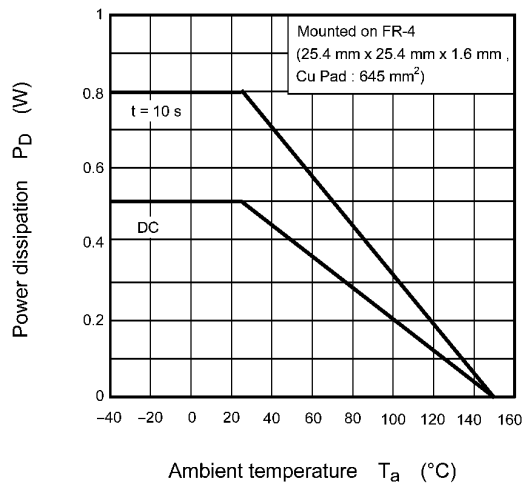
Fig. 7.1.12 P_D - T_a
