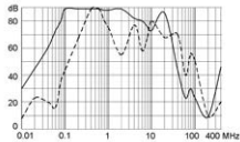
50A (FMAC-0934-5010L)
