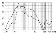
36A (FMAC-0934-3610)
