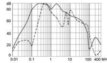
16A (FMAC-0931-1612I)
