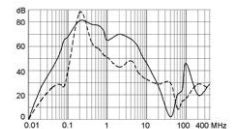
50A (FMAC-0934-5010)
