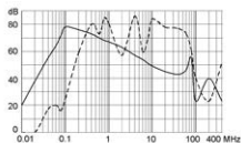
110A (FMAC-0954-H110)
