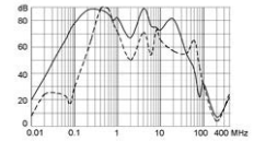
64A (FMAC-0934-6410L)
