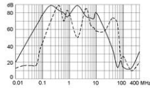
25A (FMAC-0932-2512I)
