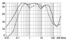
180A (FMAC-0955-H210)
