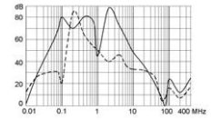
50A (FMAC-0934-5012I)
