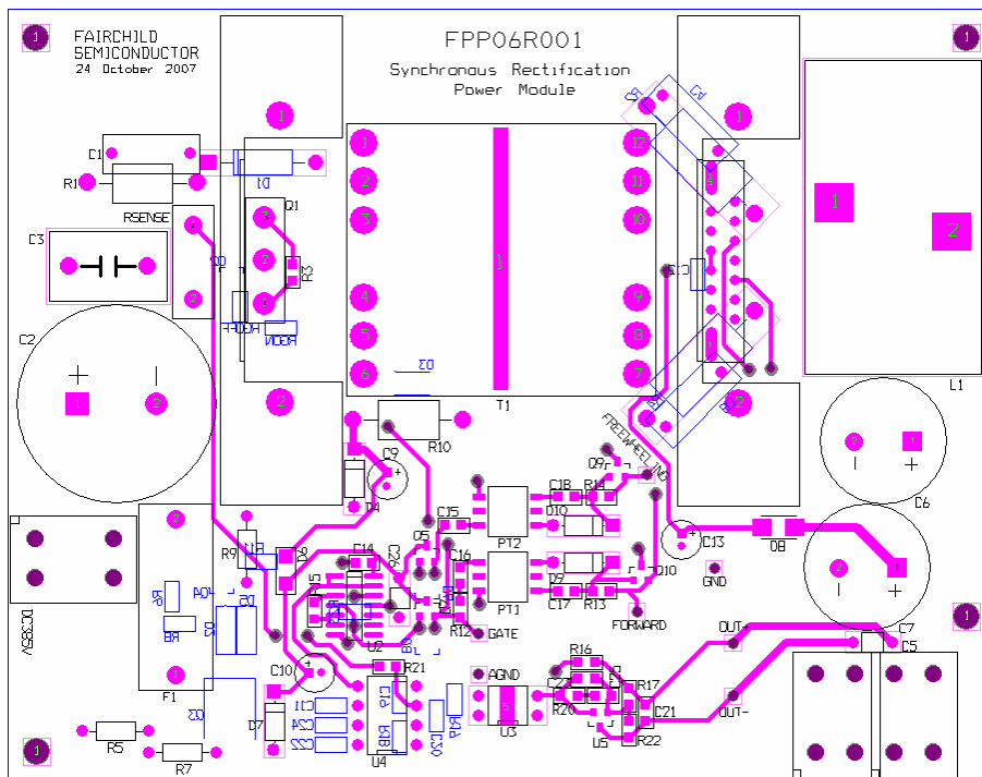
< Top layer >
