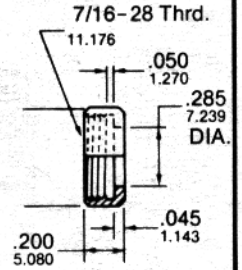
1/2" HEX NUT
