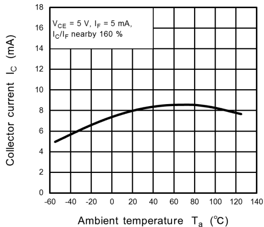
Fig. 11.13 I_C - T_a
