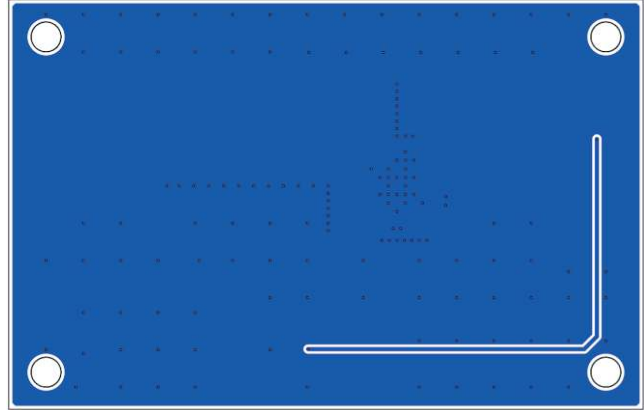
Layer 2 (Signal)
