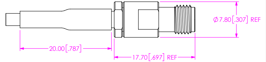
FIG 10 -92SJ SHOWN
