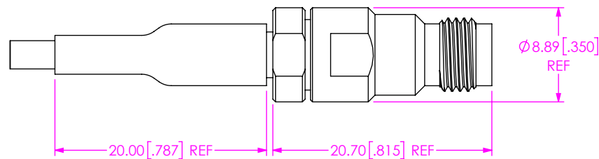
FIG 12 -24SJ SHOWN
