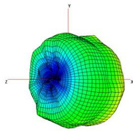
704MHz
