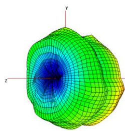
751MHz
